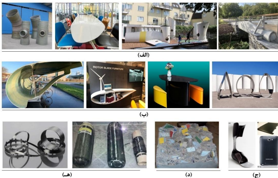
شکل ۲: بازیافت پسماندهای کامپوزیتی به روش‌های (الف) باز استفاده یا تغییر کاربری، (ب) استفاده از بخش‌هایی از سازه برای کاربری‌های مجدد، (ج) تبدیل به موادی دیگر برای سایر کاربری‌ها، (د) بازیافت برای استفاده به صورت ماده متراکم و (ه) استفاده مجدد از الیاف با کیفیت مناسب [۲۵، ۳۰، ۳۱]
